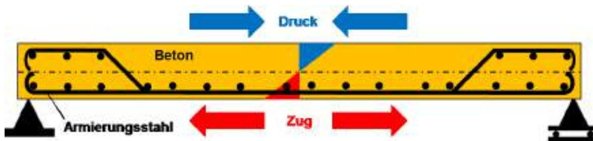
Abb. 55: Querschnitt durch eine Stahlbetondecke (stark vereinfacht)
