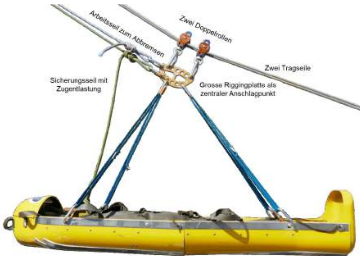
Abb. 74: Patiententransport mit einer einfachen Schrägseilbahn
