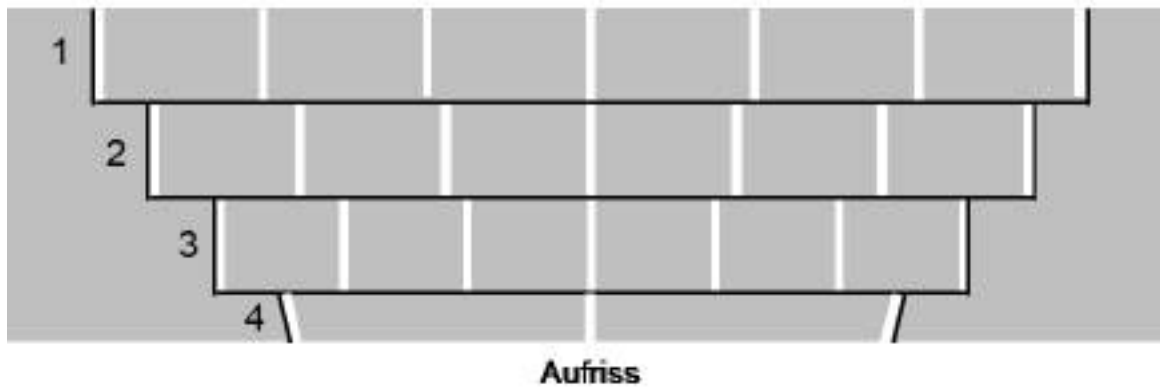
Abb. 61: Stufenschnitt-Technik
