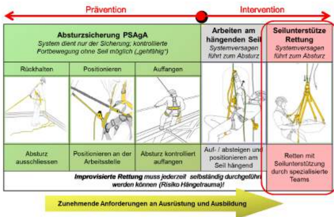
Abb. 63: Systematik Absturzsicherung – Seilunterstützte Rettung
