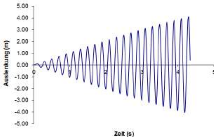
Abb. 16: Resonanz (Hans Hausammann)
