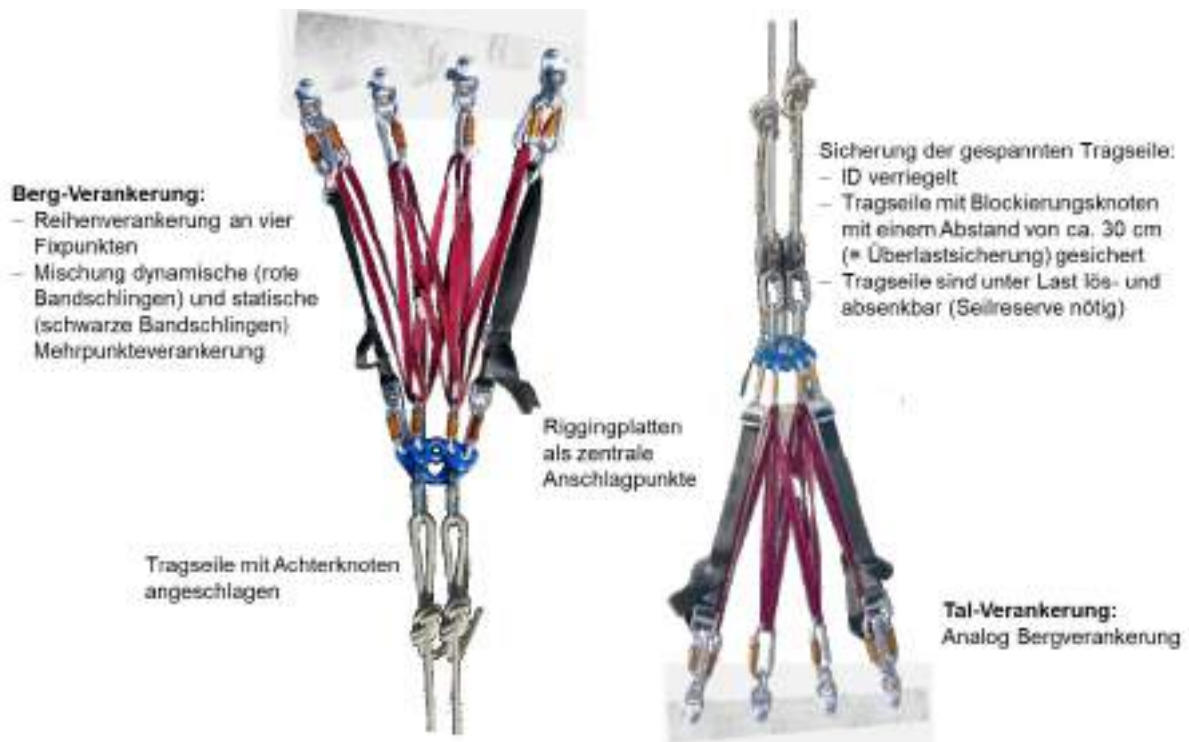
Abb. 75: Beispiel einer Berg- und Talverankerung auf Beton mit je einer Reihenverankerung an vier Fixpunkten
