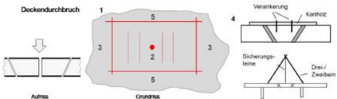
Abb. 60: Deckendurchbruch mit Diamantwerkzeugen
