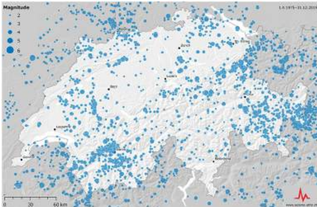
Abb. 6: Erdbebenereignisse in der Schweiz 1975–2019 (SED)
