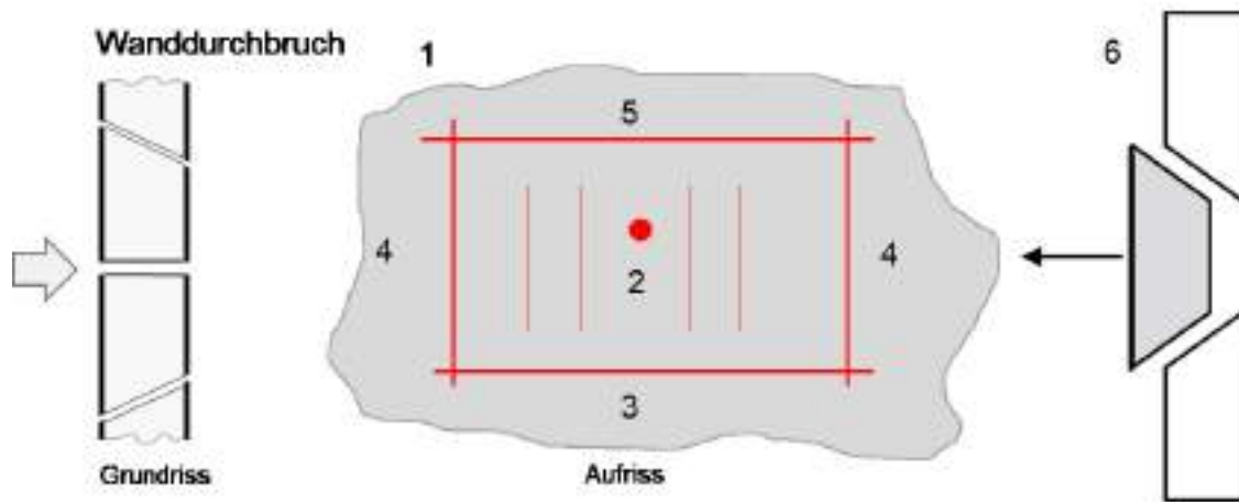
Abb. 59: Wanddurchbruch mit Diamantwerkzeugen
