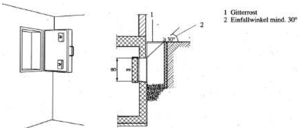
Abb. 81: Notausstieg mit Panzerdeckel und Lichtschacht
