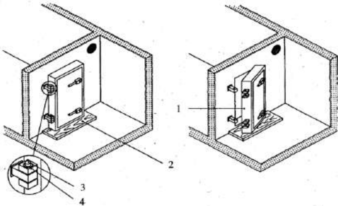
Abb. 80: Phasen beim Öffnen der Schutzraumtüre
