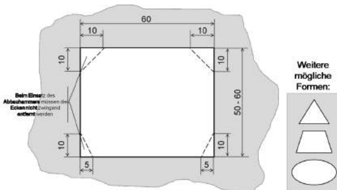
Abb. 56: Abmessung und Form eines Durchbruchs (Masse in cm)
