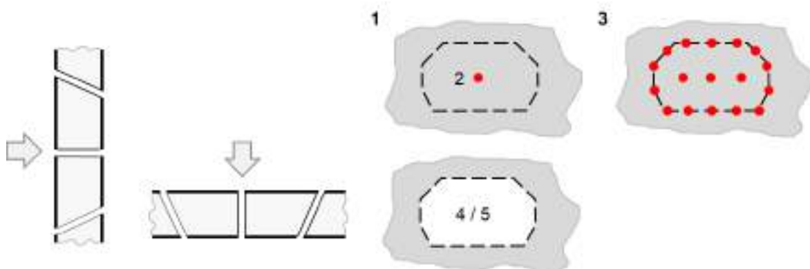
Abb. 57: Durchbrechen mit Bohr- und Abbauwerkzeugen
