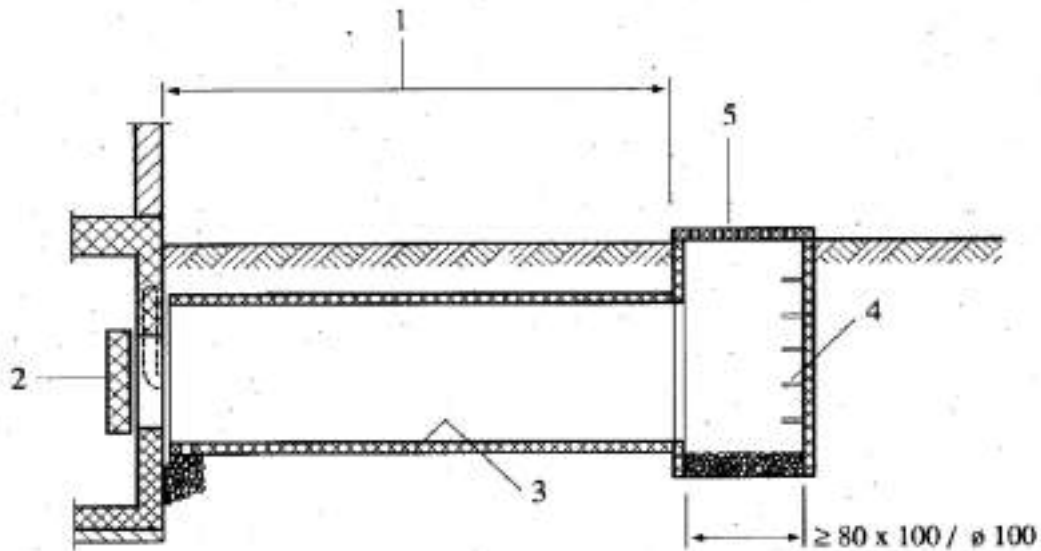
Abb. 82: Notausstieg mit Panzerdeckel, Fluchtröhre und Aufstiegschacht
