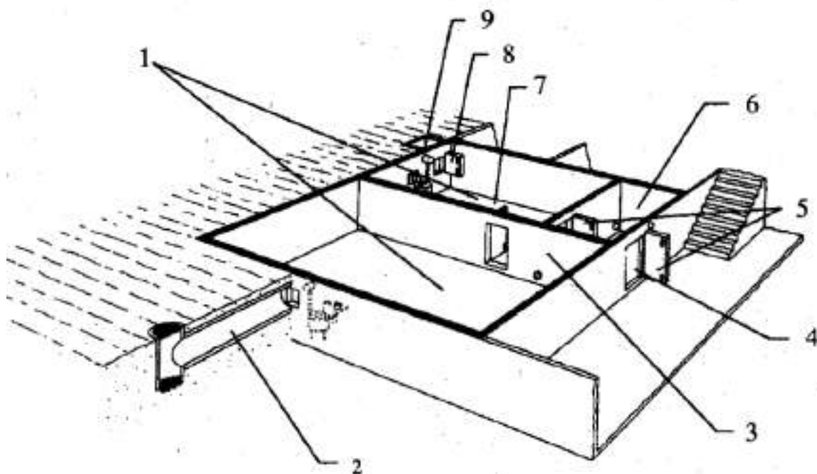
Abb. 77: Beispiel eines Schutzraums mit 51 bis 100 Schutzplätzen
