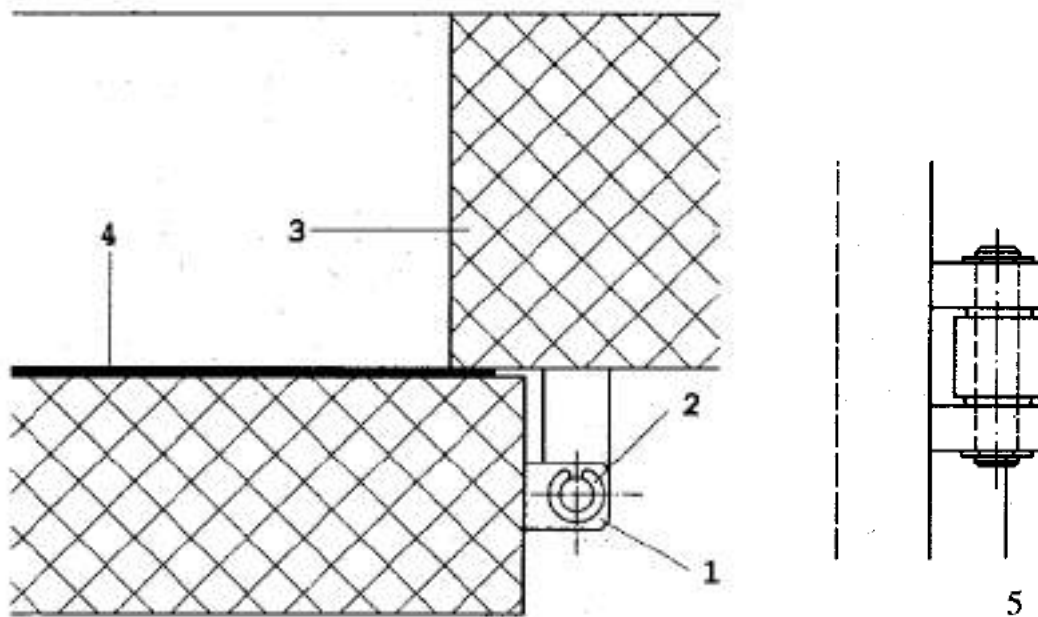
Abb. 79: Scharniere einer Panzertüre
