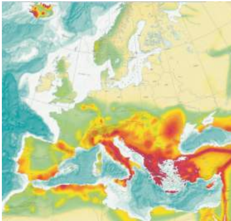
Abb. 4: Erdbebengefahr in Europa (Gardini)
