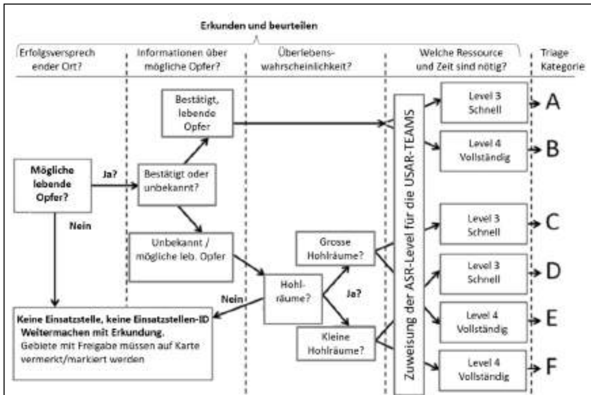
Abb. 30: Entscheidungsprozess zum Triagieren möglicher Einsatzziele (INSARAG)
