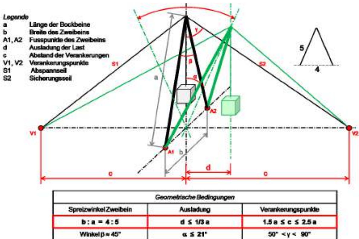
Abb. 67: Allgemeine geometrische Regeln beim Einsatz eines Zweibeins
