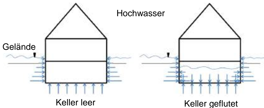
Abb. 83: Wasserdruck bei einem leeren und einem gefluteten Keller (Landesfeuerweherschule Baden-Württemberg).
