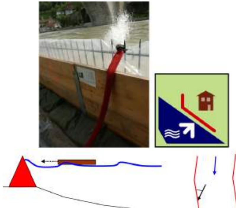
Abb. 29: Beispiel für ein System, das parallel zum Flusslauf verläuft (Vereinigung Kantonalen Feuerversicherungen VKF).
