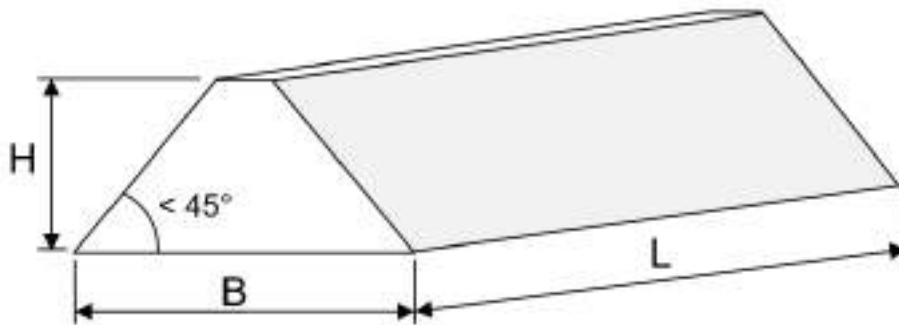
Abb. 40: Grundform eines Sandsackdamms.
