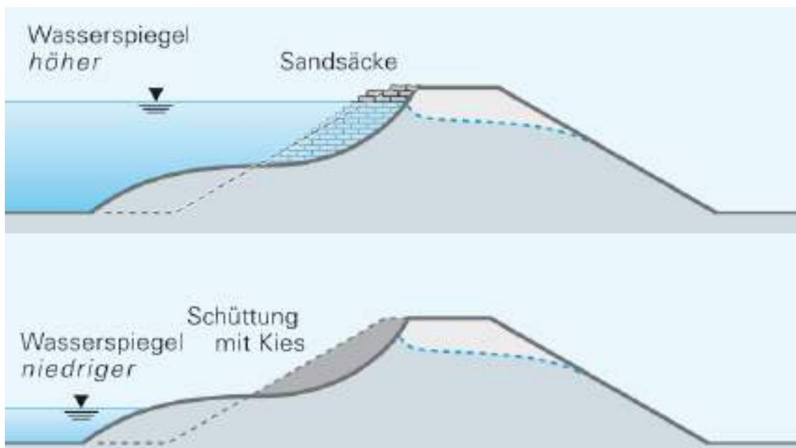
Abb. 76: Sichern von wasserseitigen Rutschungen mit Sandsäcken oder Kies (Bayerisches Landesamt für Umwelt).
